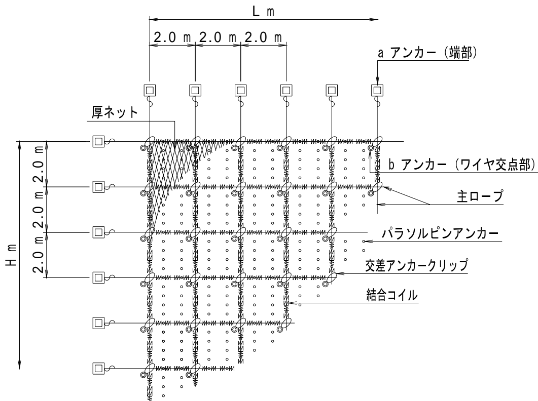
図 7 - 1 . 構造図
