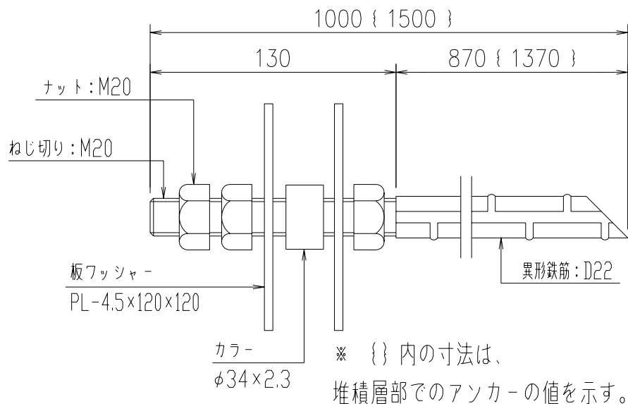
図 - 8 - 7 - 1 . 岩部用・堆積層部用 端部アンカ -
