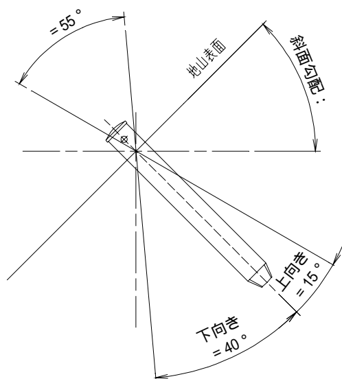
図8 - 3 - 1 . 角度管理参考モデル
