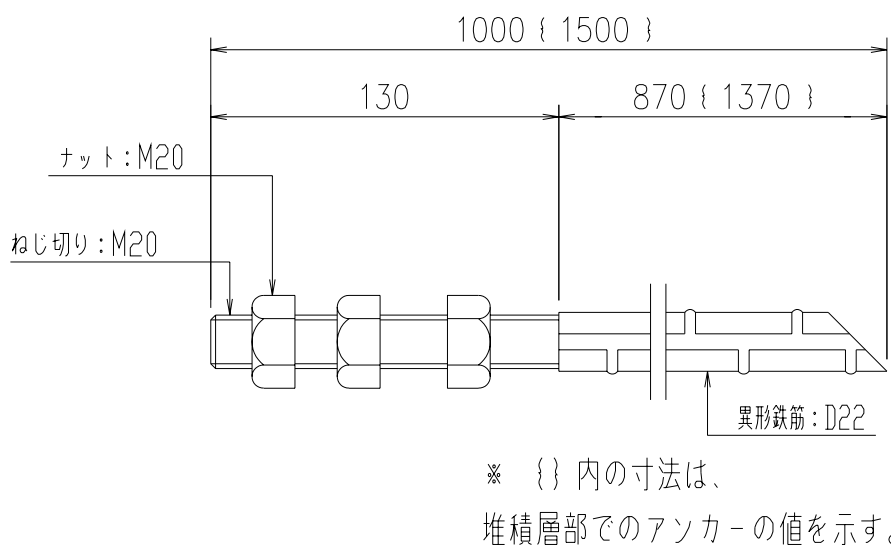
図 - 8 - 7 - 2 . 岩部用・堆積層部用 交点部アンカ -
