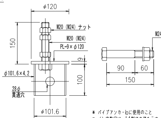
図 - 8 - 7 - 4 . 土中部用交点部アンカ -
